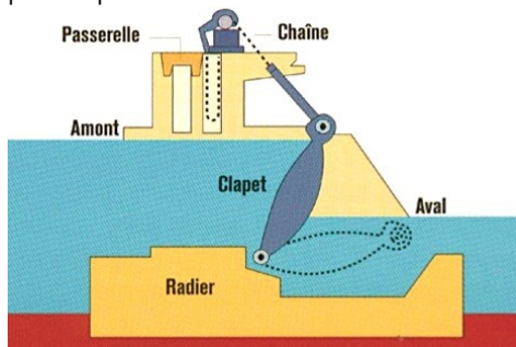
Schéma d'une vanne-clapet
